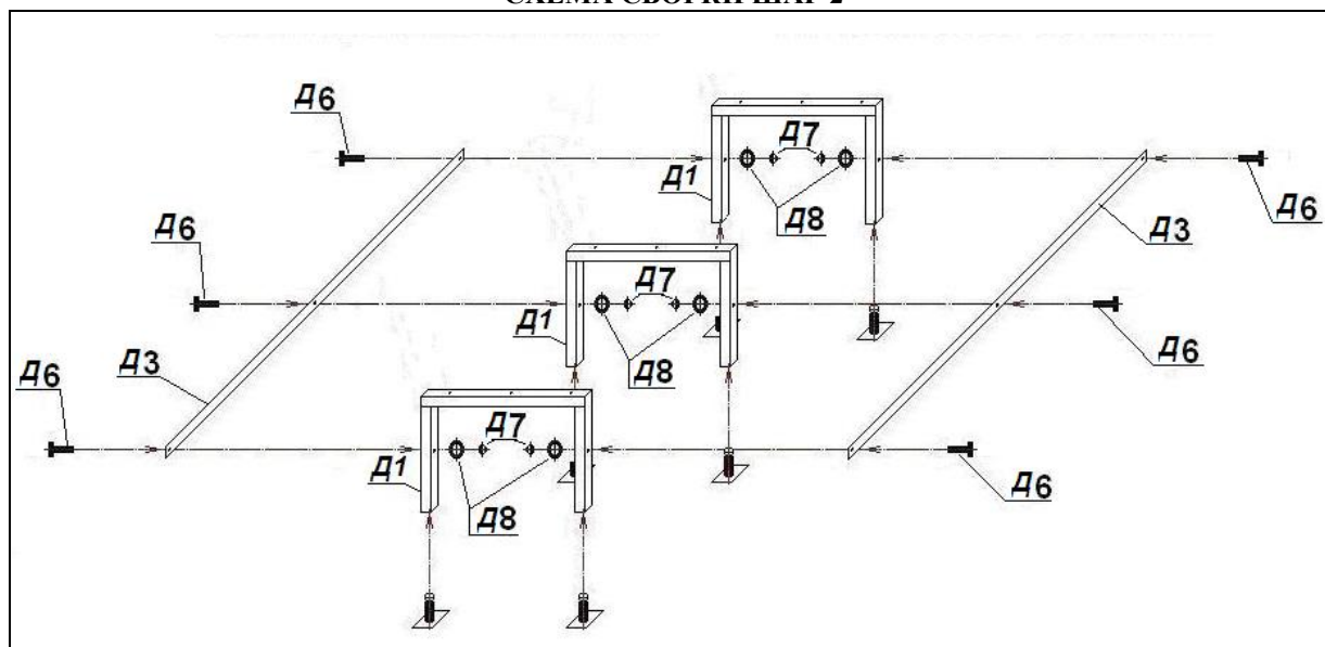
СХЕМА СБОРКИ ШАГ 2
